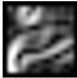
Edge Detection
